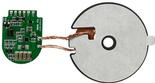
Module Front Side 模組前面
