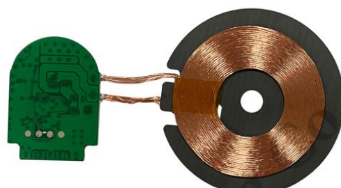
Module Back Side 模組後面
