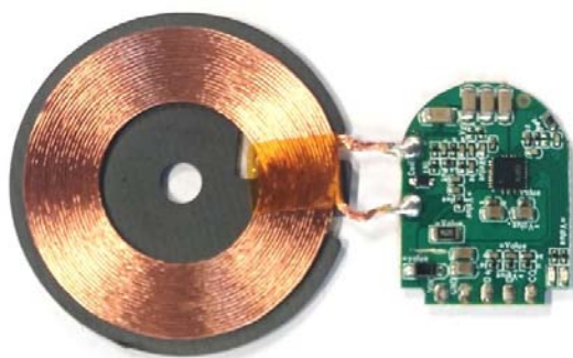
Module Front Side 模組前面
