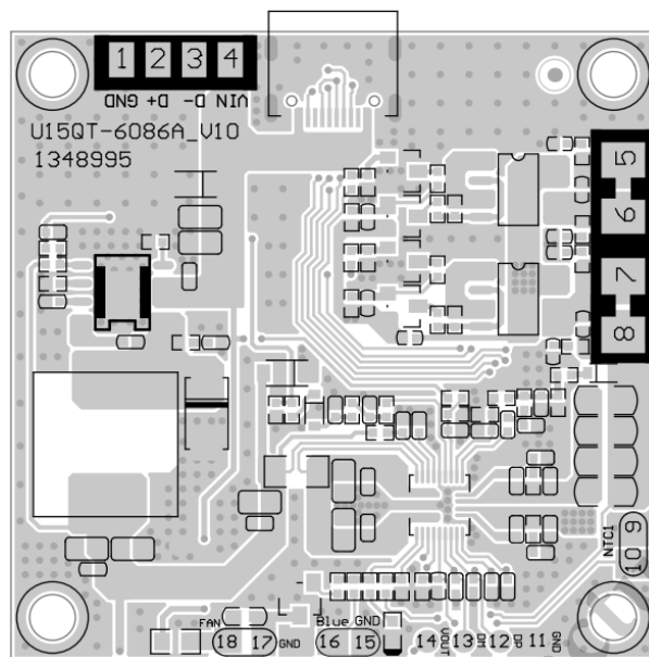
PCBA圖
