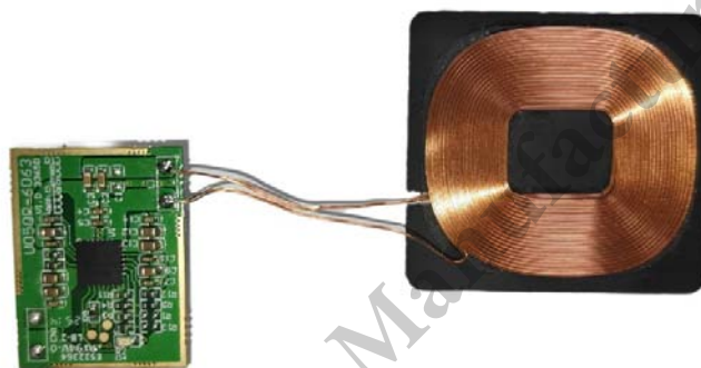
Module Front Side 模組前面
