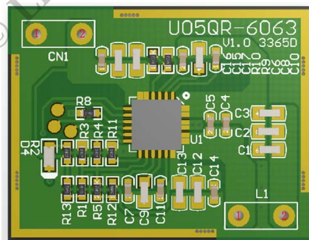
PCBA圖
