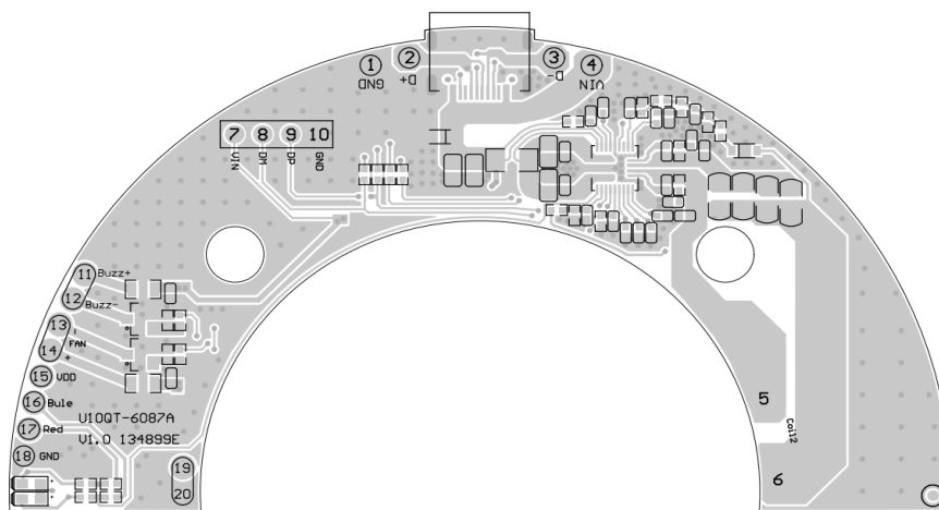
PCBA 圖
